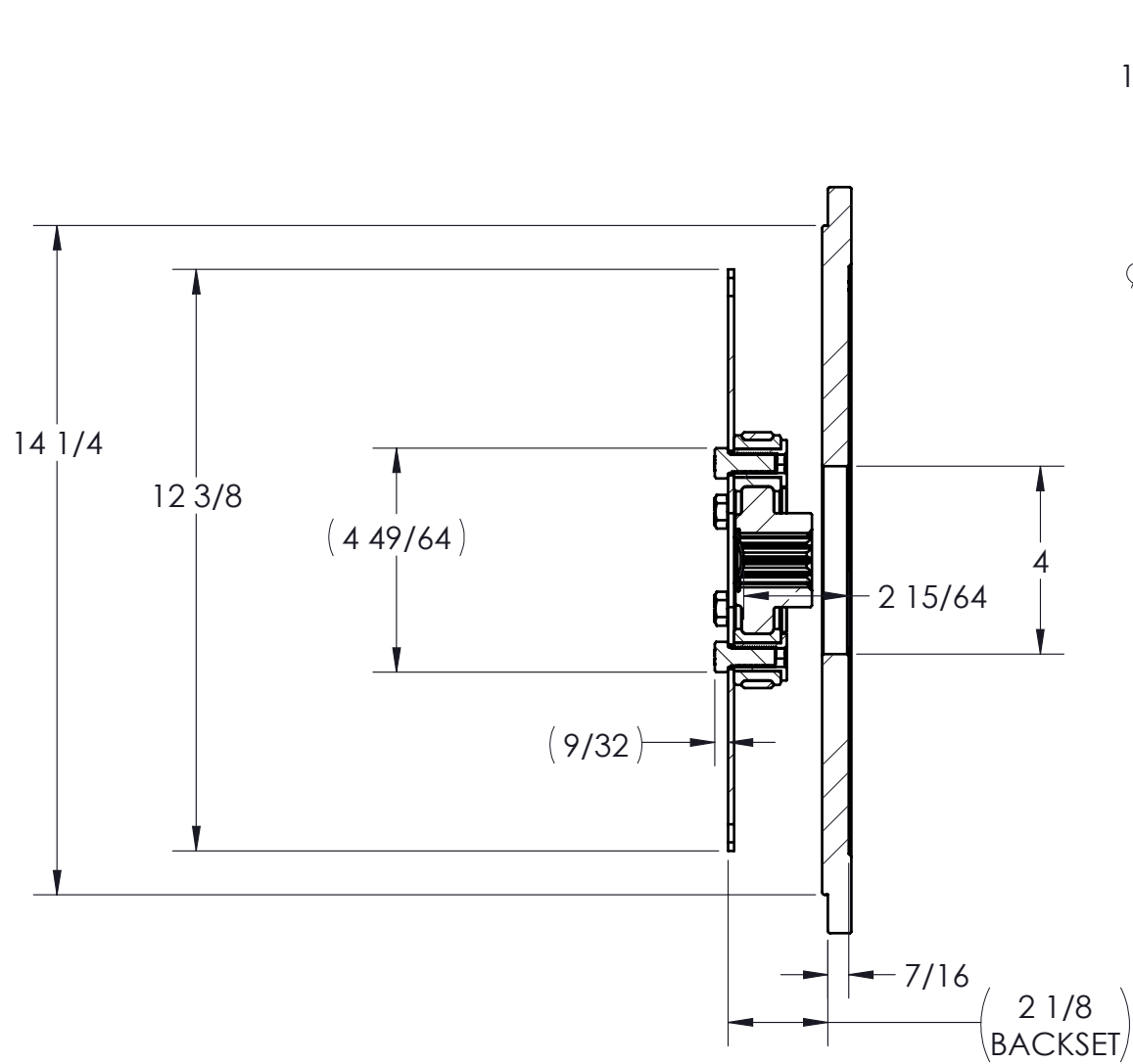
SECTION B-B SCALE 1 : 4
