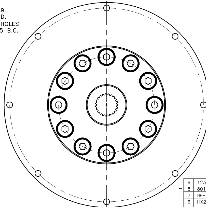
COUPLING ASS'Y PN 125995
