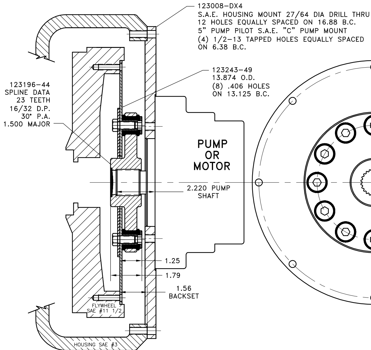
COUPLING ASS'Y PN 125995
